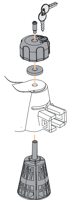
TCT000212 Cono de fijación. Conical coupling.
